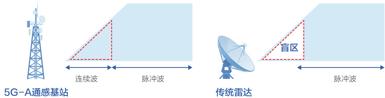
▲ 图3.4 “脉冲波+连续波”双波形感知技术原理
