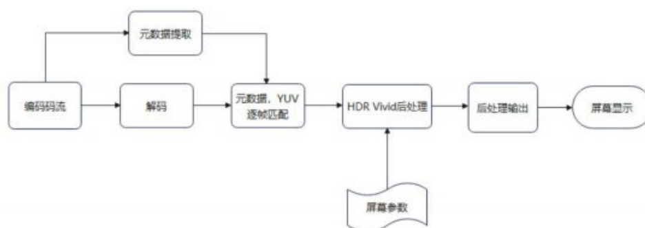
图 75 菁彩 HDR 解码显示流程
