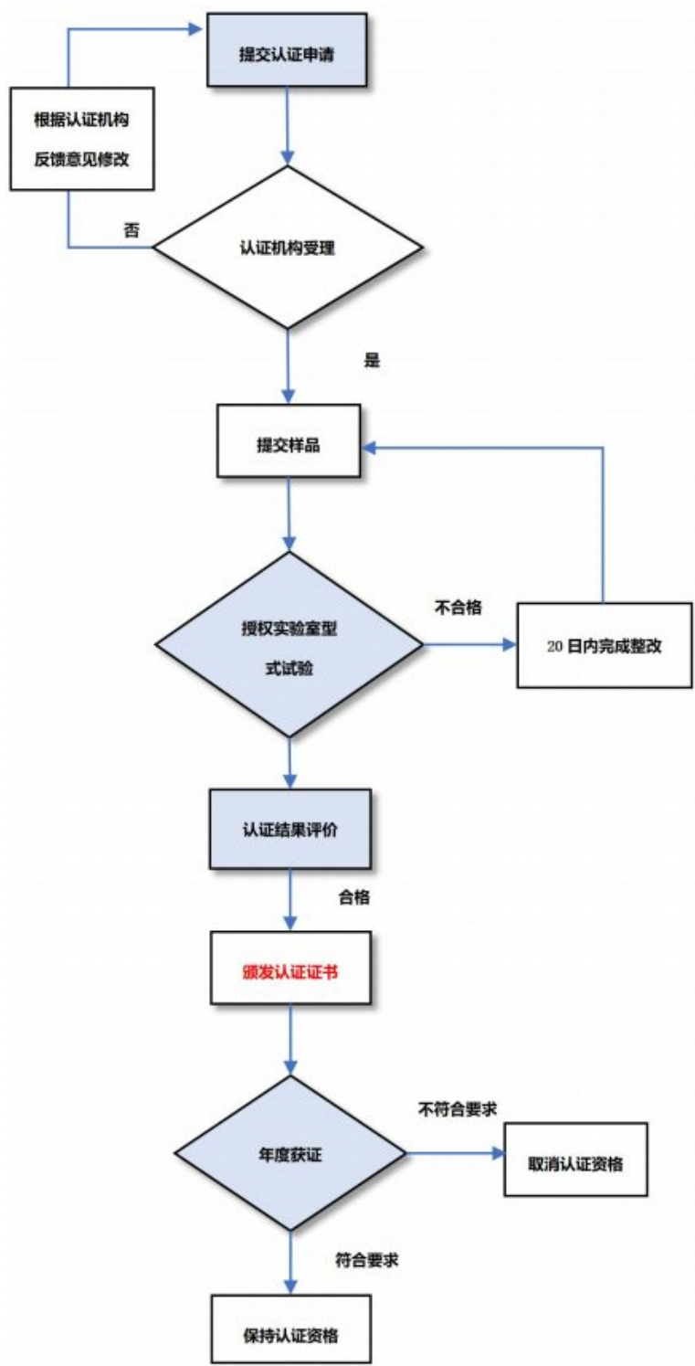
图 76 认证流程
