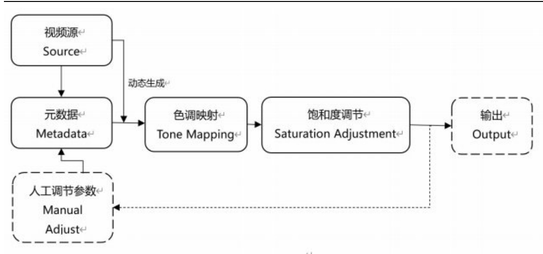
图 2 菁彩 HDR 技术原理分解
