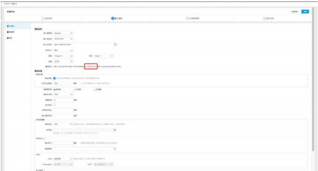
图 51 HLG 输入源
