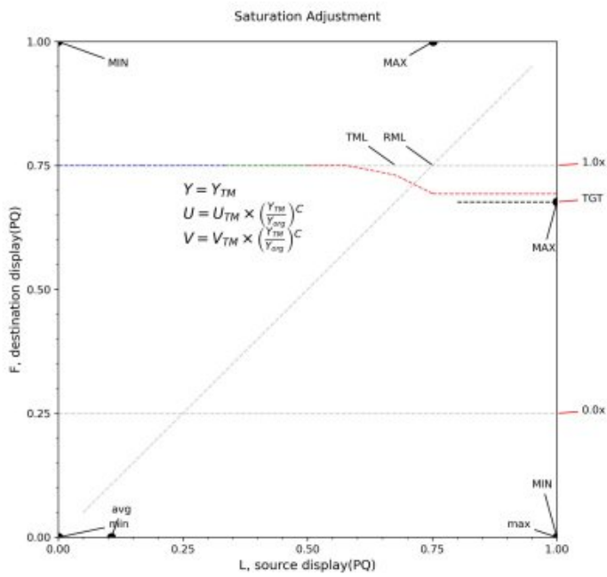
图 4 饱和度调整
