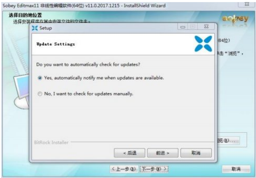
图 19 安装设置
