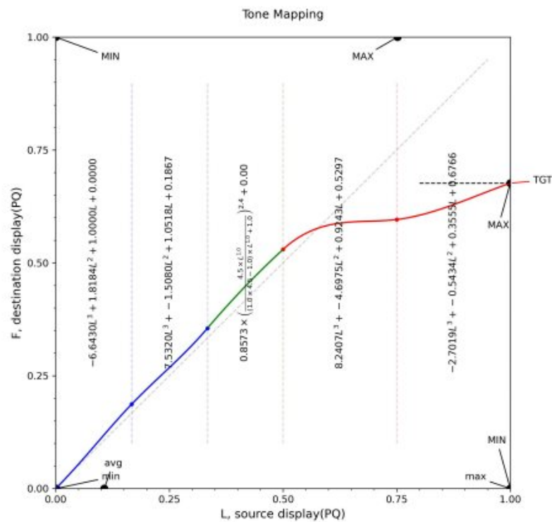
图 3 元数据映射
