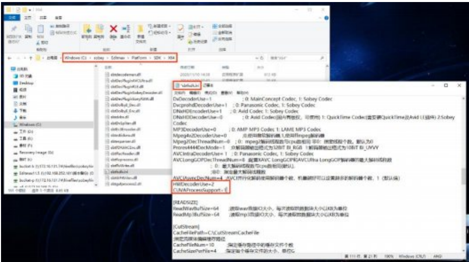
图 24 脚本设置
