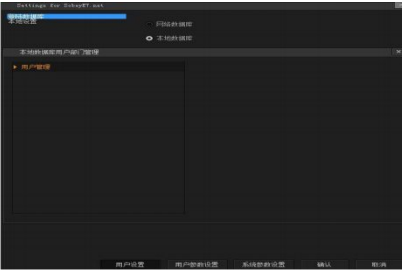
图 23 登录设置
