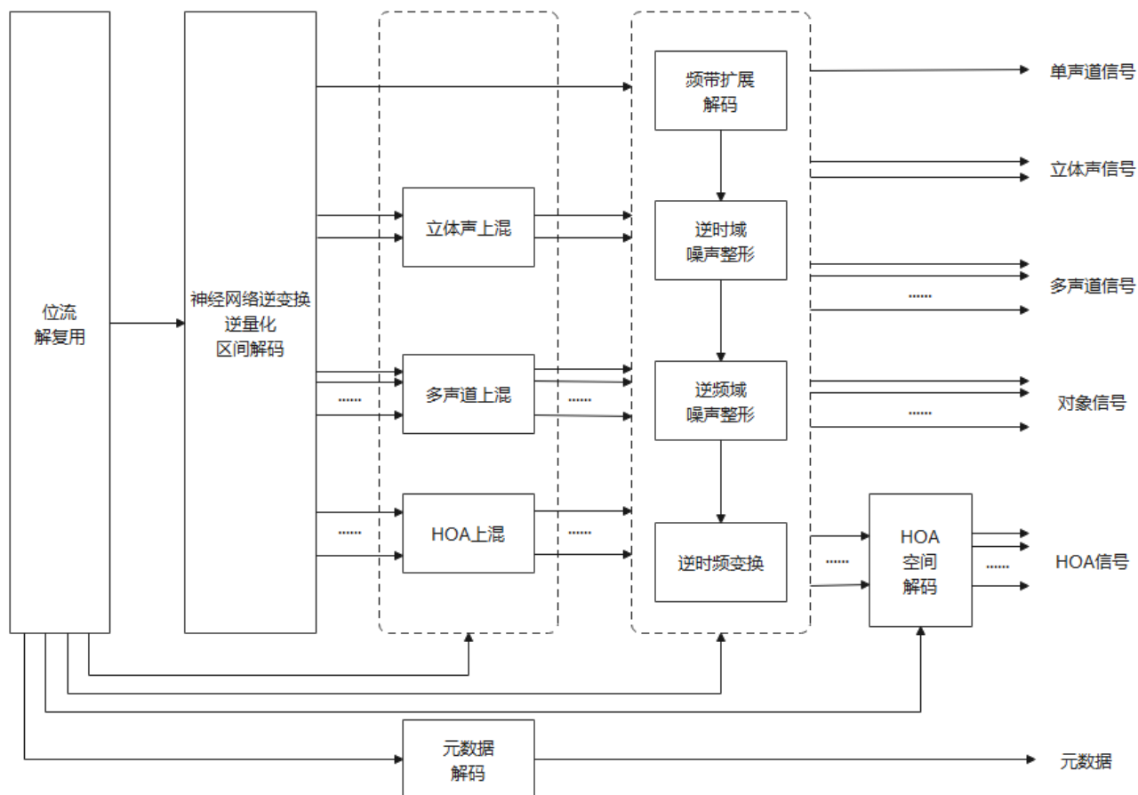
图 6 通用全码率音频解码器框架
