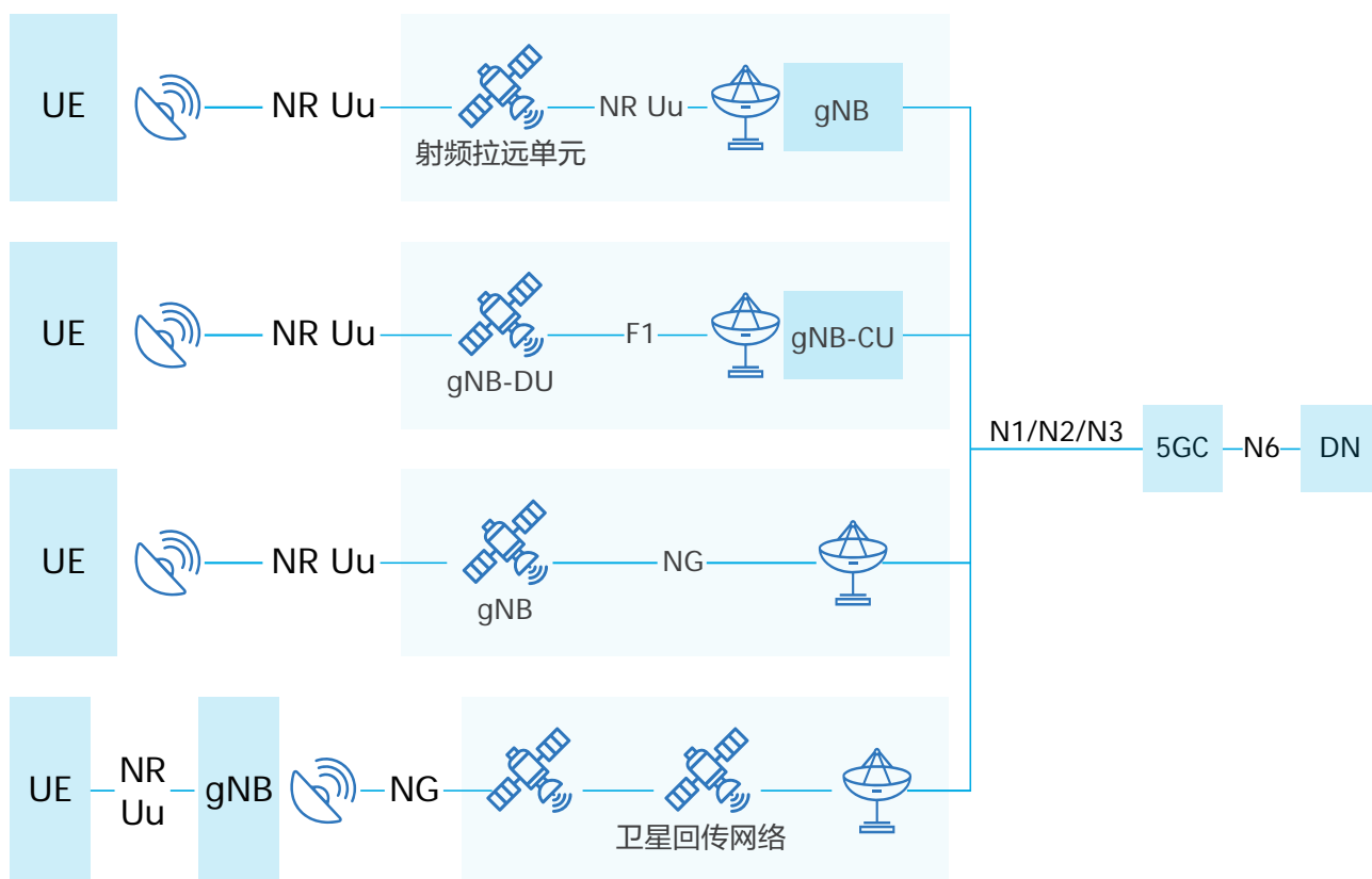
图 3.4-1：融合卫星系统的 5G 网络
