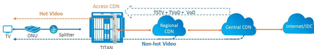
图 5-1 OLT 内置刀片实现 Access CDN
