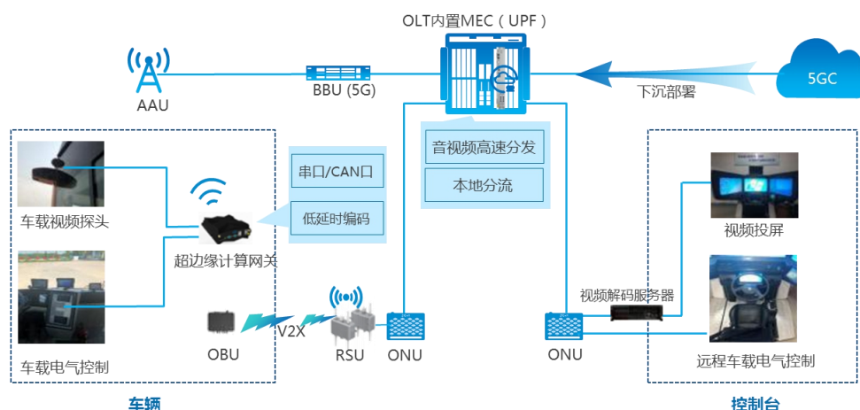
图 5- 5 OLT 内置刀片支持远程驾驶
